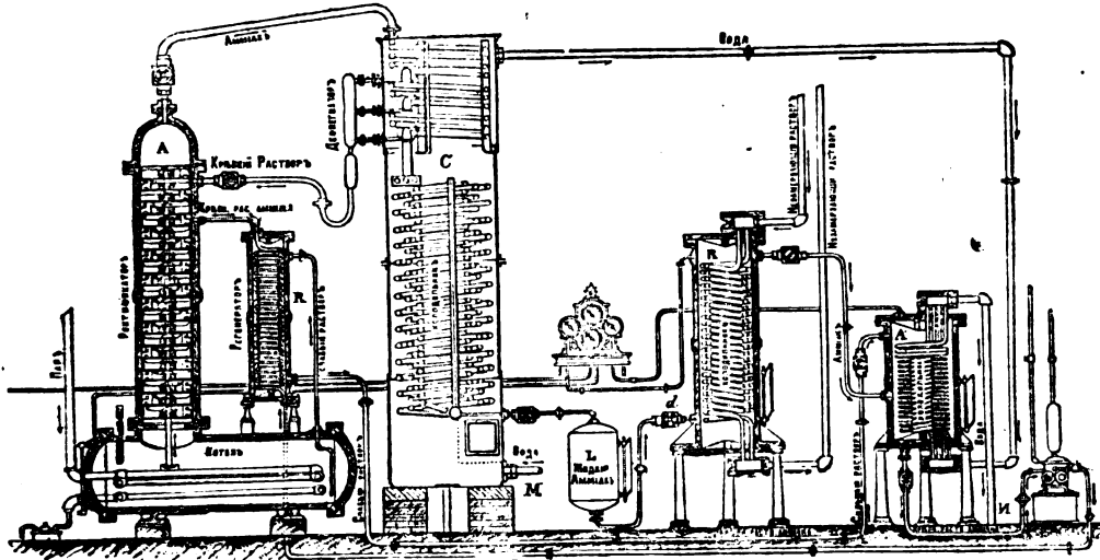
Фиг. 2. Абсорбціонная амміачная машина Понтифенса и Вуда. Система Карре.
